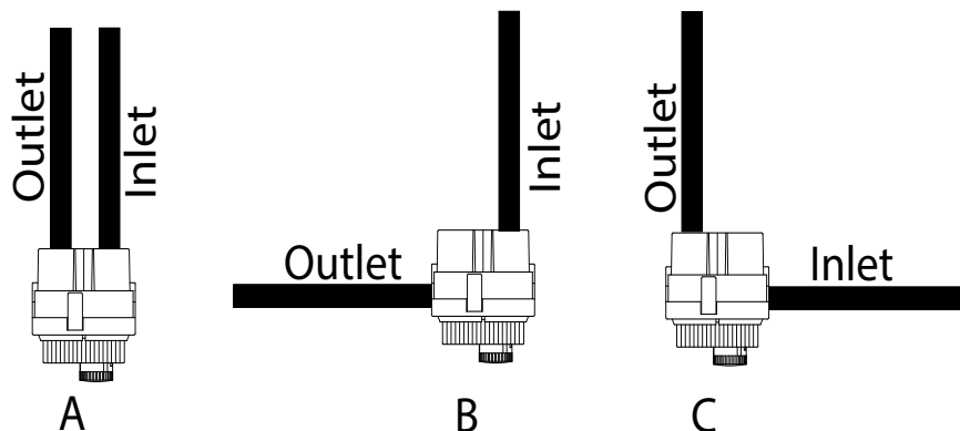
Fig. 3 Plumbing options
